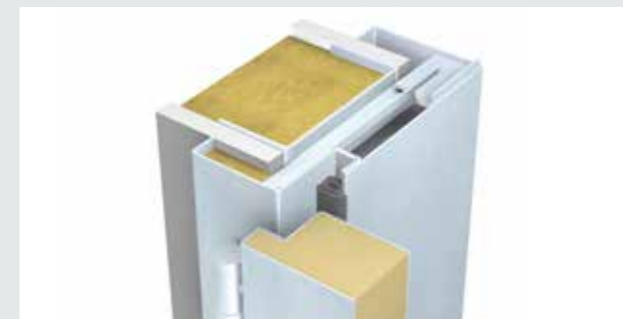
Das bewährte Prinzip der 2-schaligen Zargen für den nachträglichen Einbau
