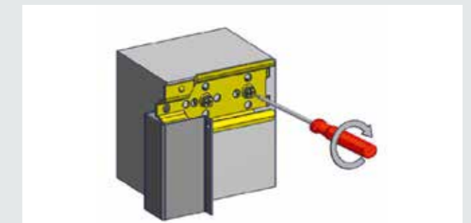
Der Nivellieranker mit Führungsanker ist besonders montagefreundlich. Mit einem Schraubendreher lässt sich der Abstand zur Wand einfach einstellen.
