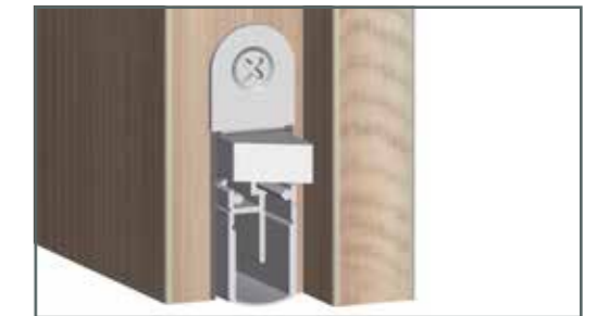
Die mechanisch absenkbare Bodendichtung hindert Schall und Zugluft.
