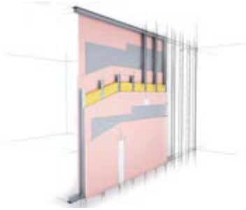
Brandwände / Brandschutz bis 90 Minuten Feuerwiderstand mit zusätzlicher mechanischer Beanspruchung
